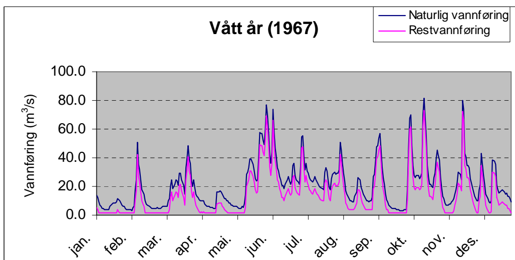
Figur 2. Vassføringskurver for Etneelva nedstrøms Stordalsvatnet før (blå strek) og etter regulering (raud strek) for eit tørt år (eksempel 1960), for eit middels år (eksempel 1978) og for eit vått år (eksempel 1967).
